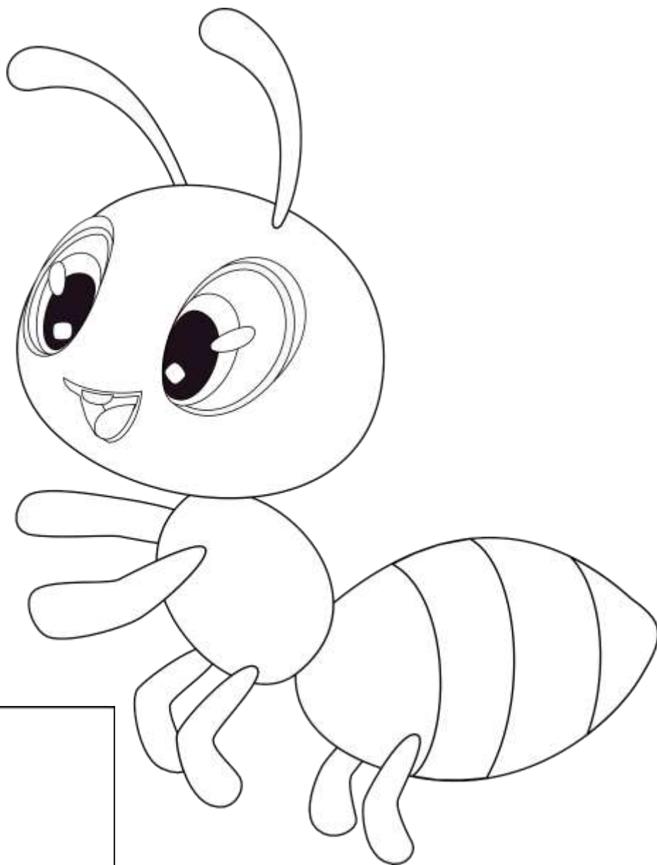
Ant
